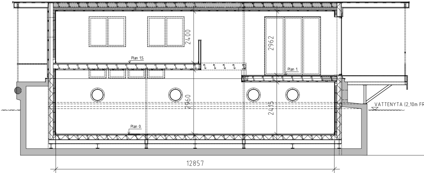
Längdsektion, longitudinal section
