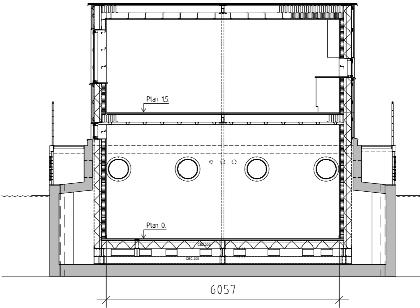
Tvärektion, cross section
