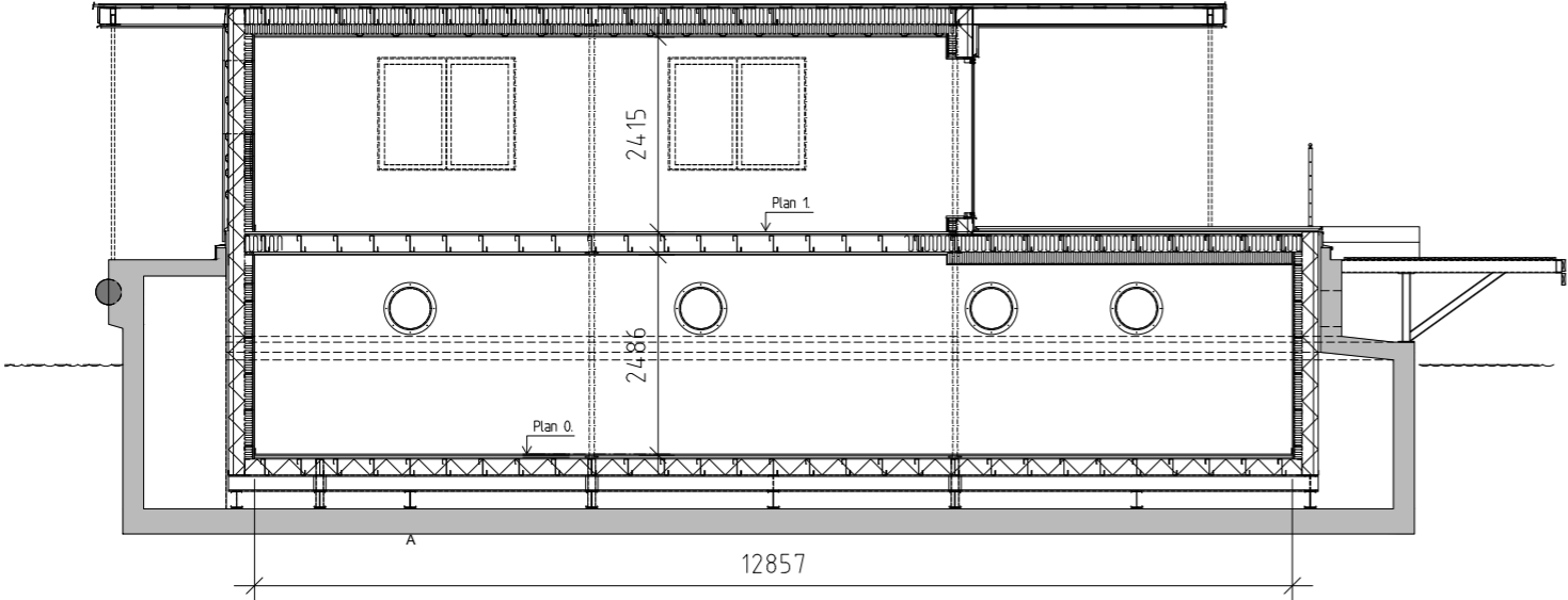
Längdsektion, longitudinal section
