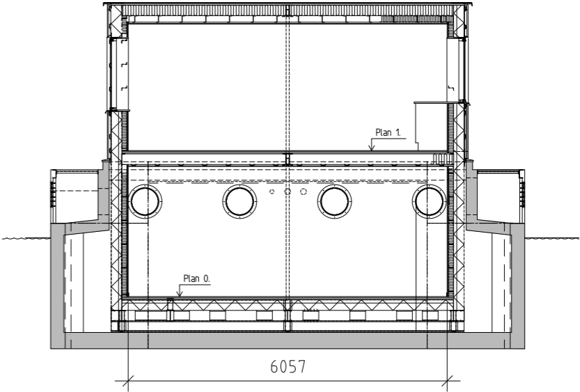
Tvärsektion, cross section
