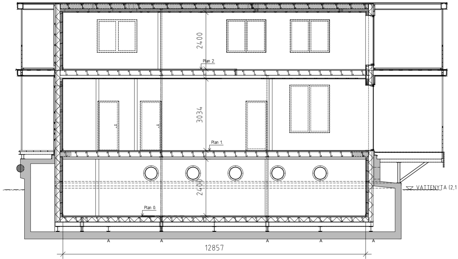
Längdsektion, longitudinal section
