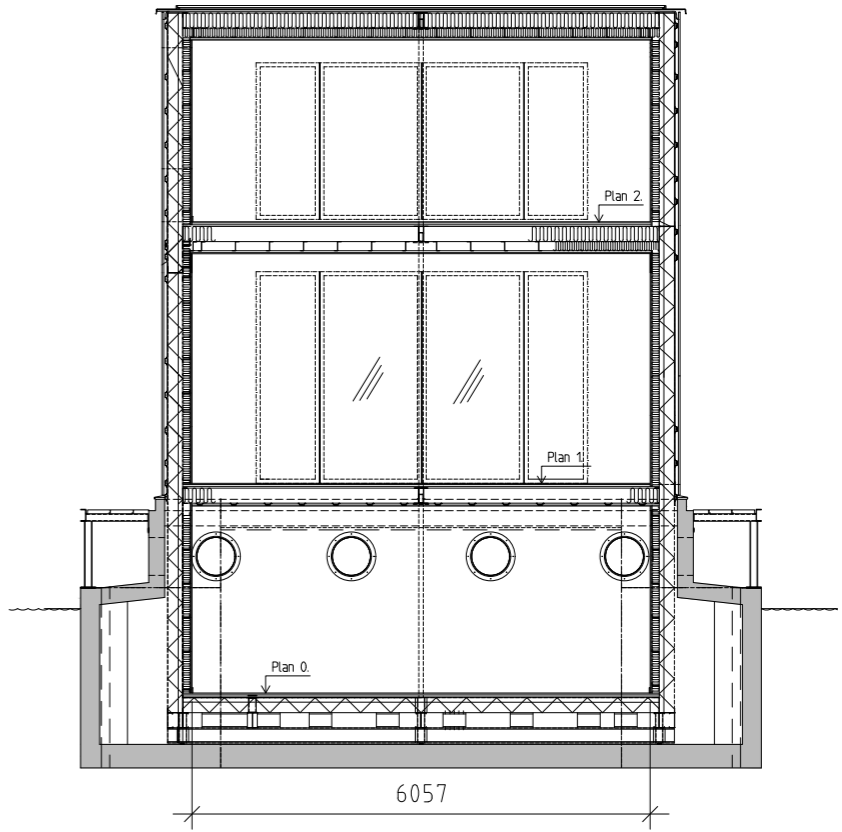
Tvärsektion, cross section
