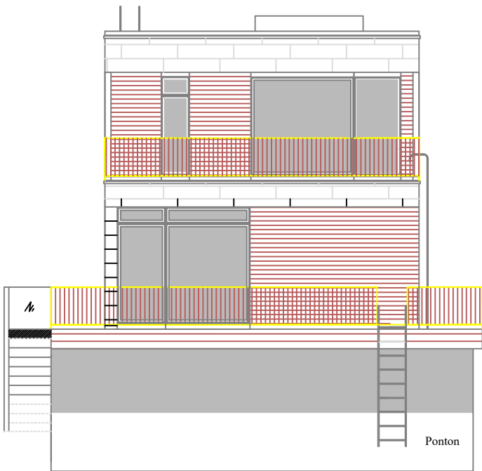
FASAD - AKTER
